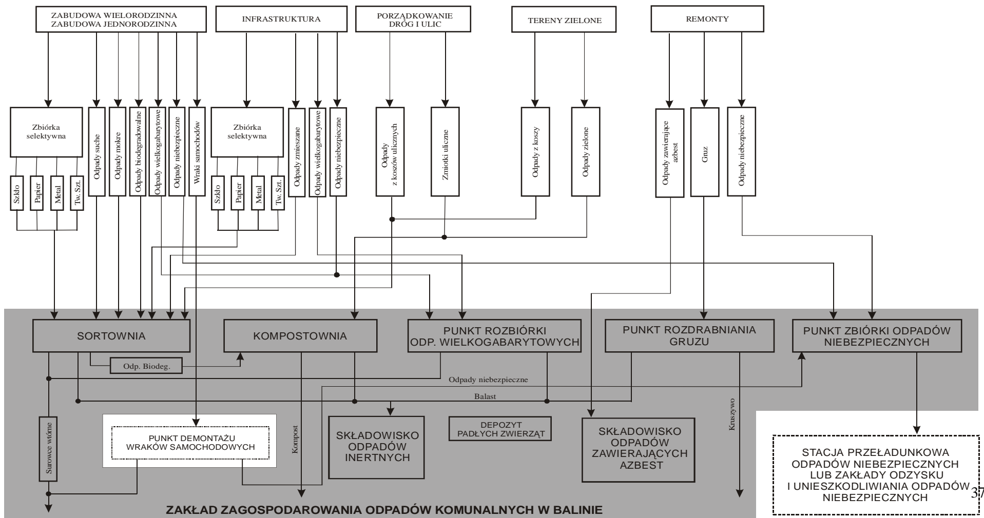
Rys. 3.5.1. System gospodarki odpadami komunalnymi dla gminy Babice w oparciu o Zakład Zagospodarowania Odpadów w Balinie (wprowadzenie systemu wielopojemnikowego dla zabudowy jednorodzinnej, surowców wtórnych, odpadów niebezpiecznych, wielkogabarytowych i budowlanych)
